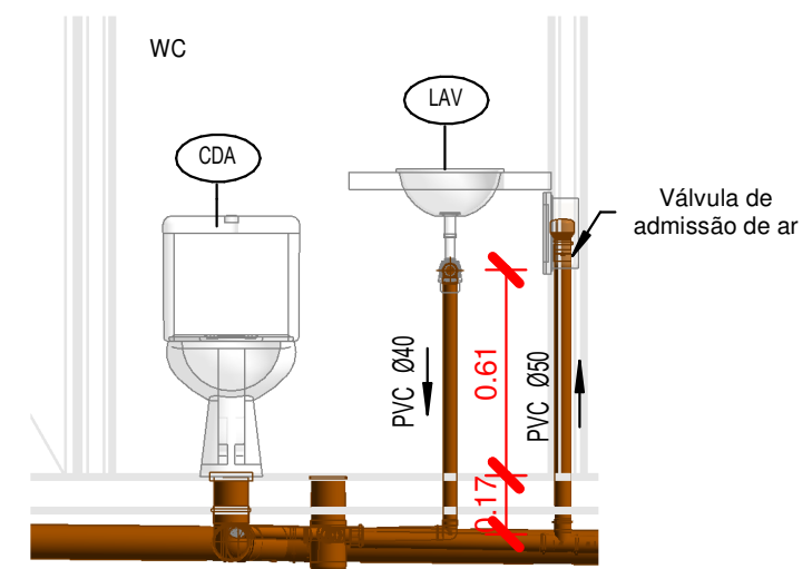
VISTA 03 - ESGOTO 1 : 25
