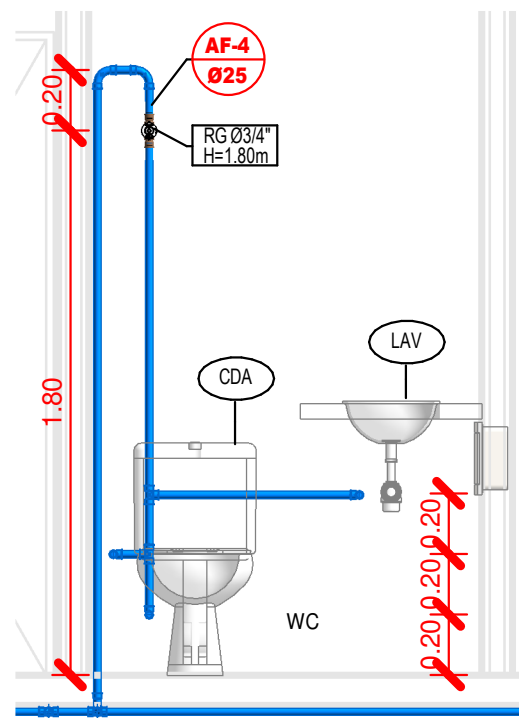
VISTA 03 - ÁGUA FRIA 1 : 25
