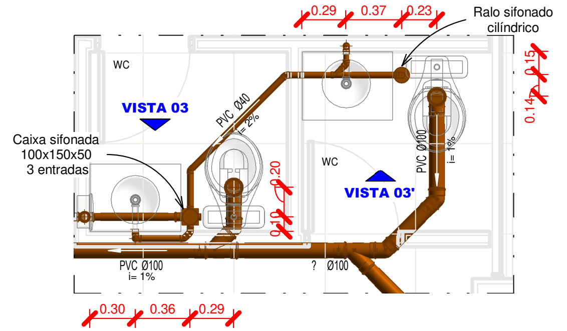
DETALHE 03 - ESGOTO 1 : 25
