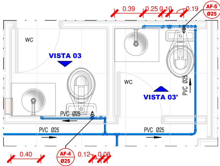
DETALHE 03 - ÁGUA FRIA 1 : 25
